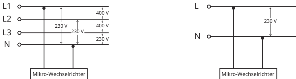
Abbildung 1-6 Unterstützte Netztypen
